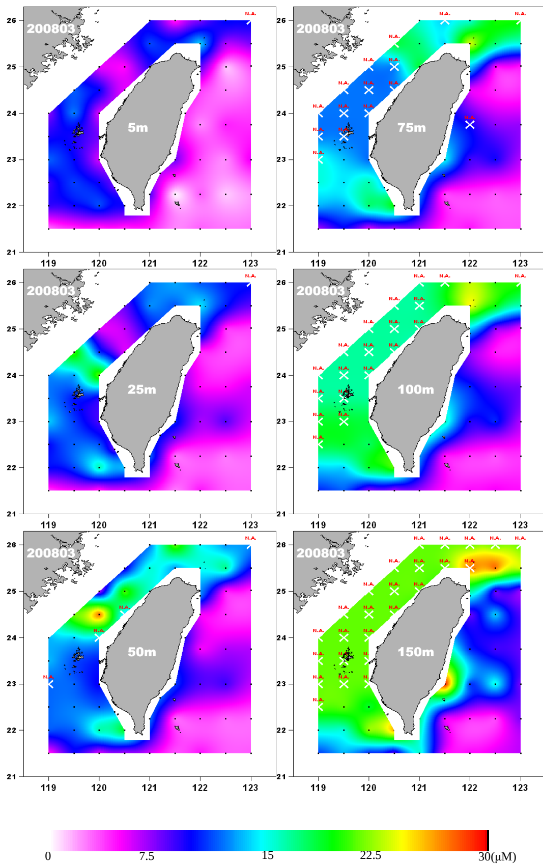
圖 22. 2008-03-13 航次矽酸鹽( \text{SiO}_4 )濃度分布 Fig. 22. Silicate ( \text{SiO}_4 ) distribution in Mar. 2008.
