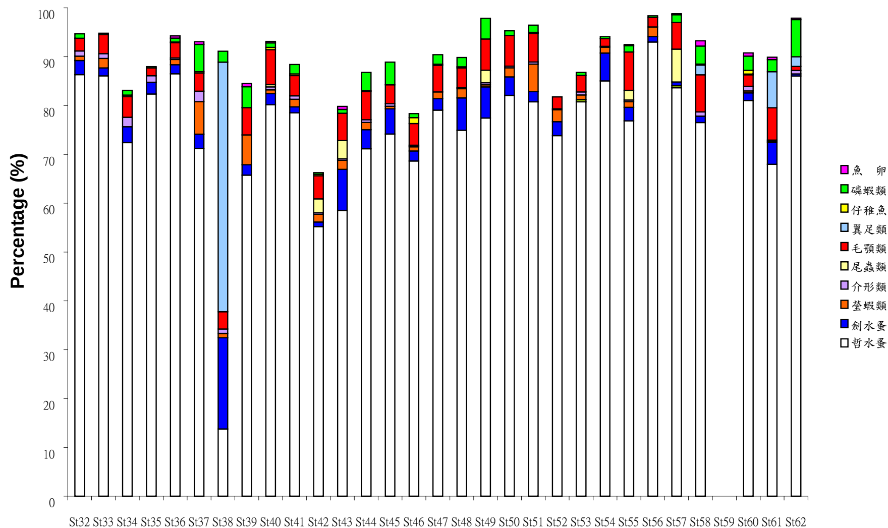
圖 35. 2008-03-13 航次浮游動物優勢大類出現百分率
