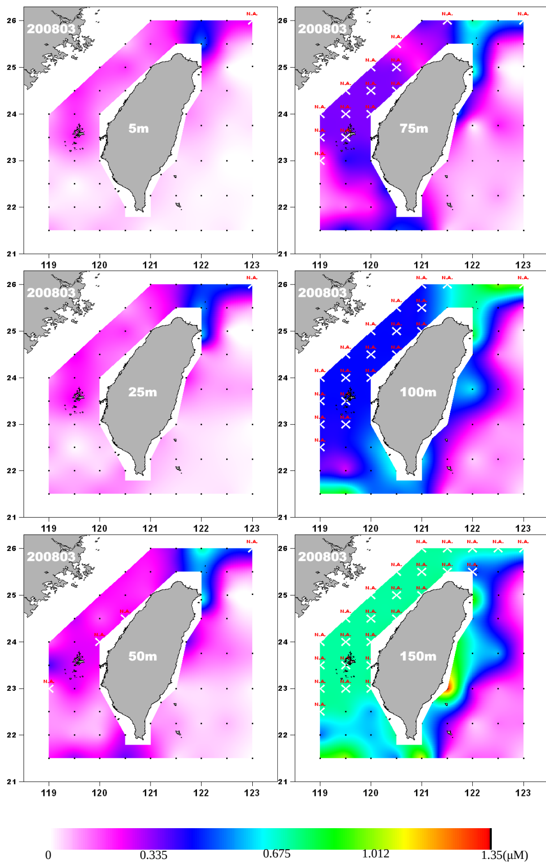
圖 18. 2008-03-13 航次磷酸鹽( \text{PO}_4 )濃度分布 Fig. 18. Phosphate ( \text{PO}_4 ) distribution in Mar. 2008.
