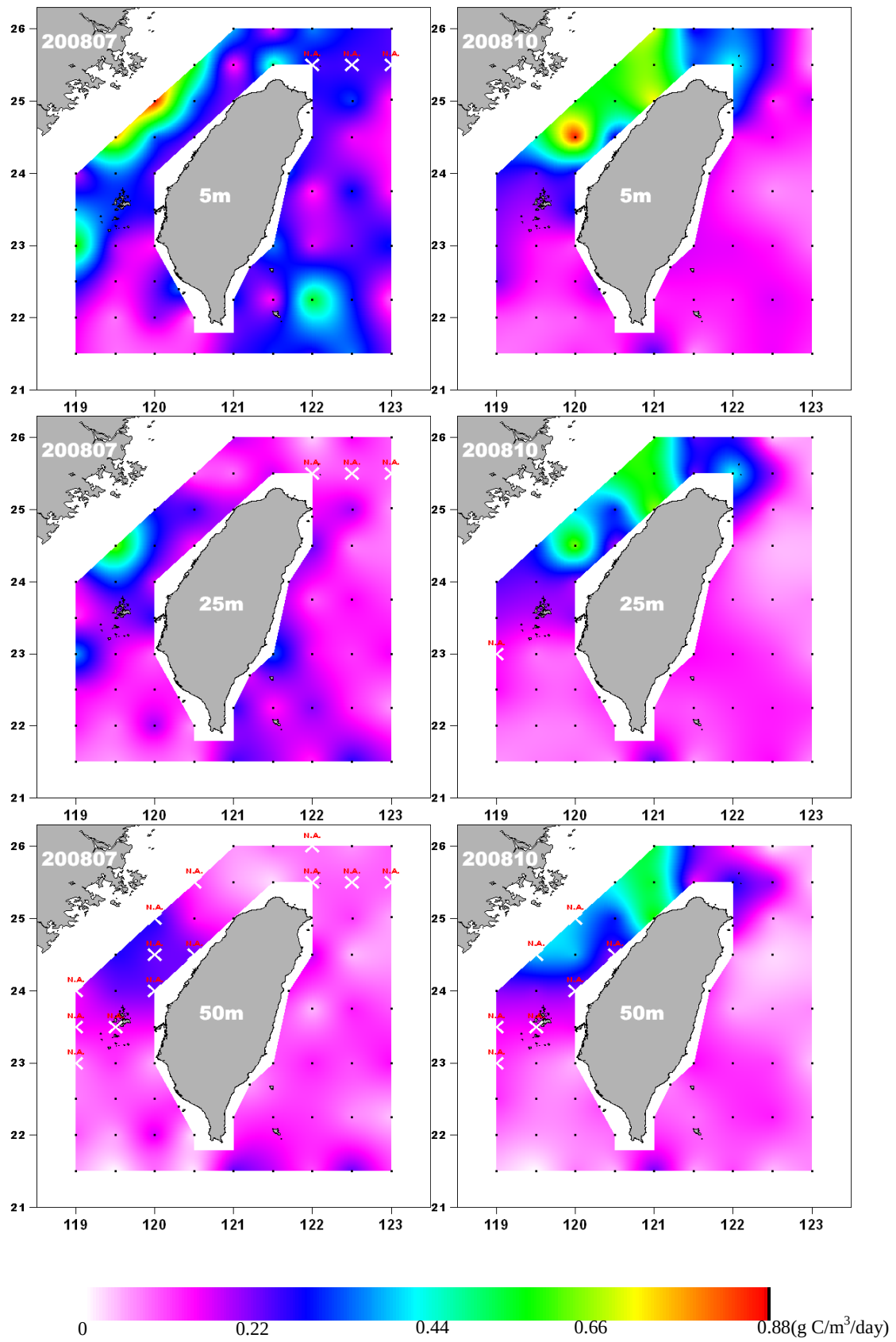
圖 30. 2008 年 7 月及 10 月基礎生產力分布 Fig. 30. Primary production distribution in Jul. and Oct. 2008.
