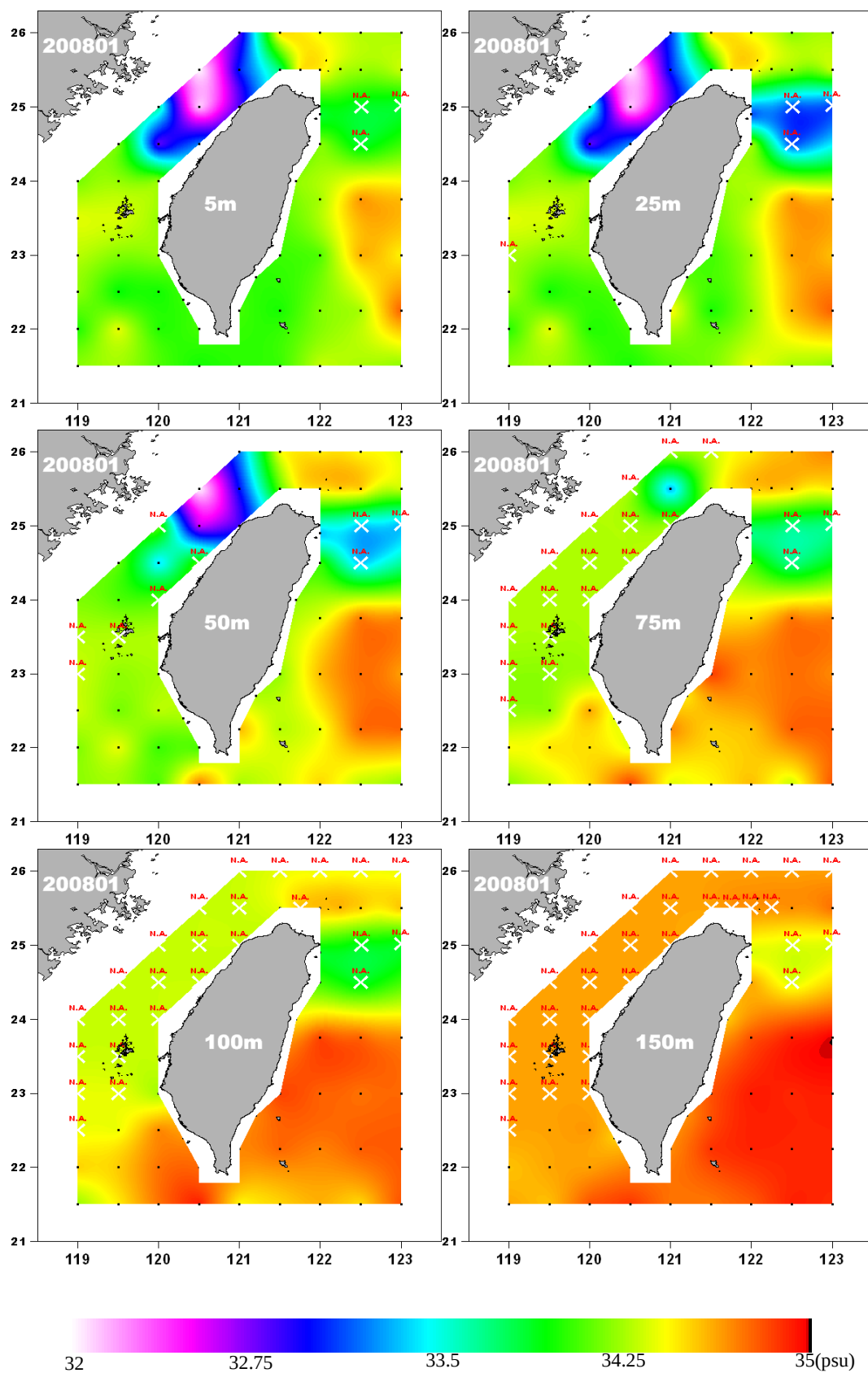
圖 9. 2008-01-04 航次鹽度分布 Fig. 9. Salinity distribution in Jan. 2008.
