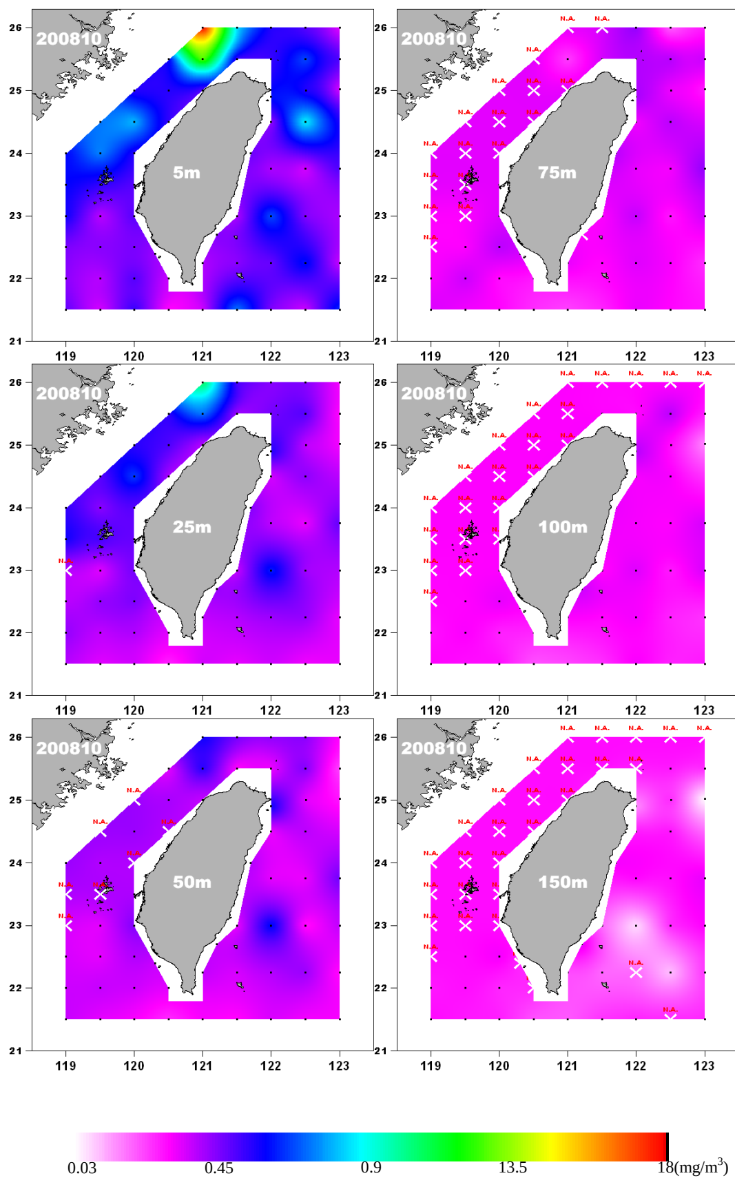
圖 28. 2008-10-14 航次葉綠素甲(chl-a)濃度分布 Fig. 28. chlorophyll(chl-a) distribution in Oct. 2008.
