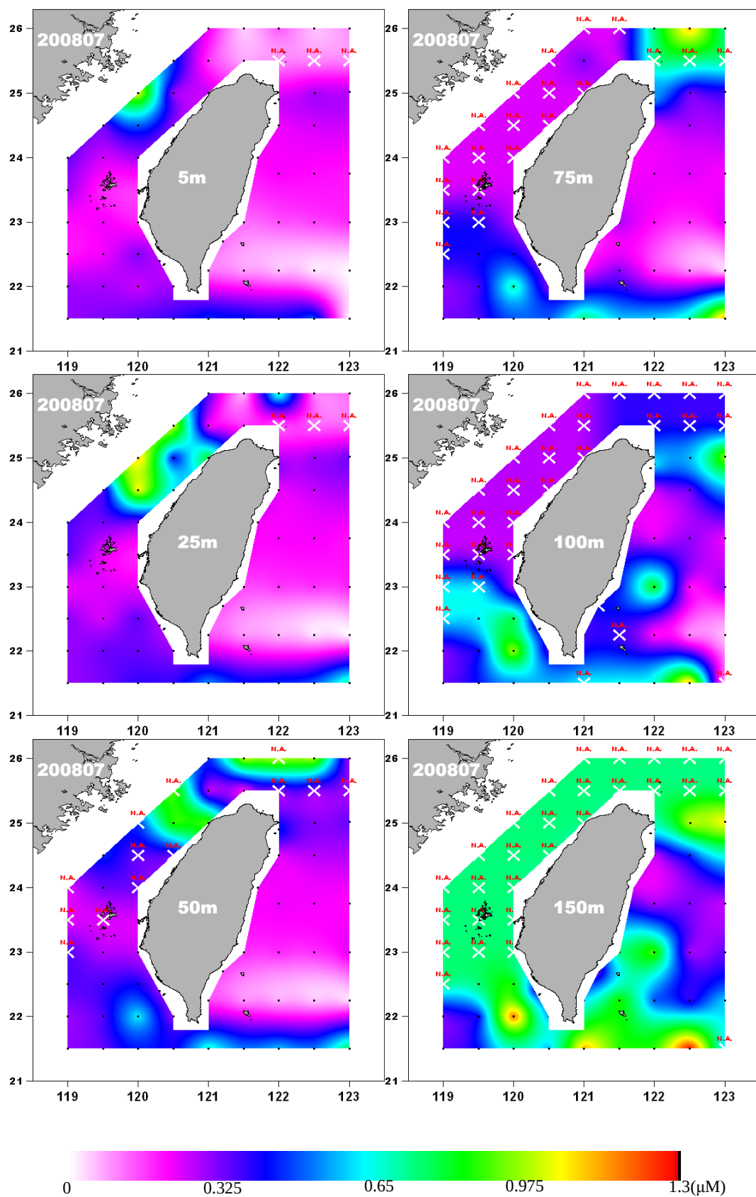
圖 19. 2008-07-03 航次磷酸鹽( \text{PO}_4 )濃度分布 Fig. 19. Phosphate ( \text{PO}_4 ) distribution in Jul. 2008.
