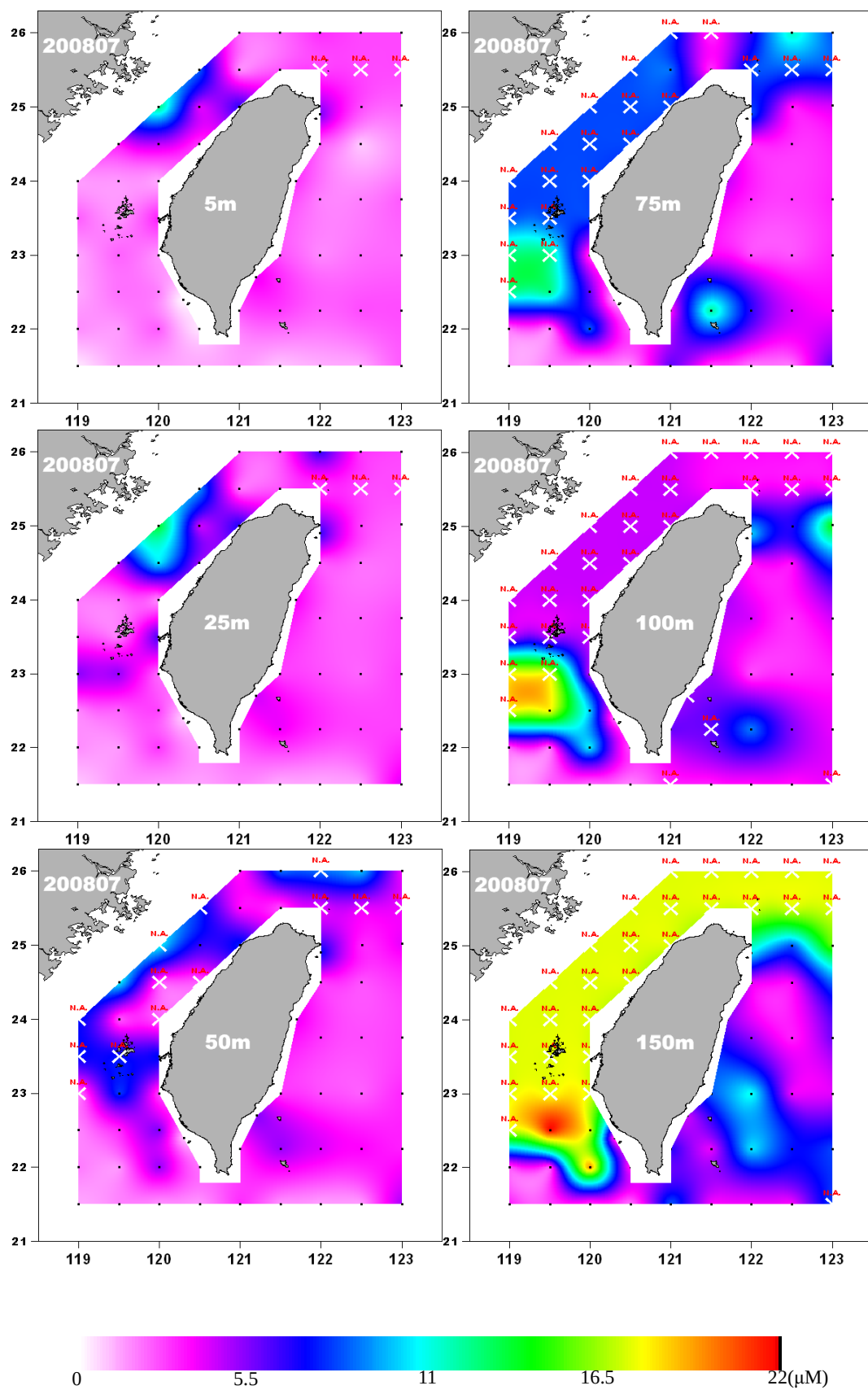
圖 23. 2008-07-03 航次矽酸鹽( \text{SiO}_4 )濃度分布 Fig. 23. Silicate ( \text{SiO}_4 ) distribution in Jul. 2008.
