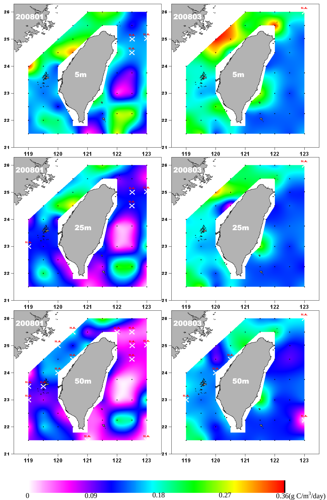
圖 29. 2008 年 1 月及 3 月基礎生產力分布
