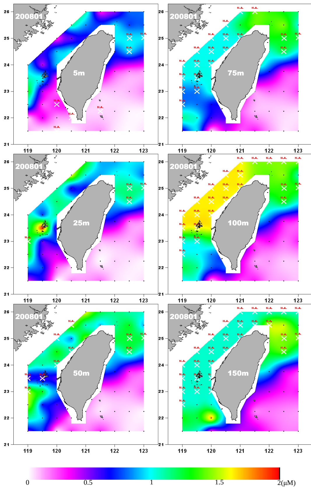
圖 17. 2008-01-04 航次磷酸鹽( \text{PO}_4 )濃度分布 Fig. 17. Phosphate ( \text{PO}_4 ) data in Jan. 2008.
