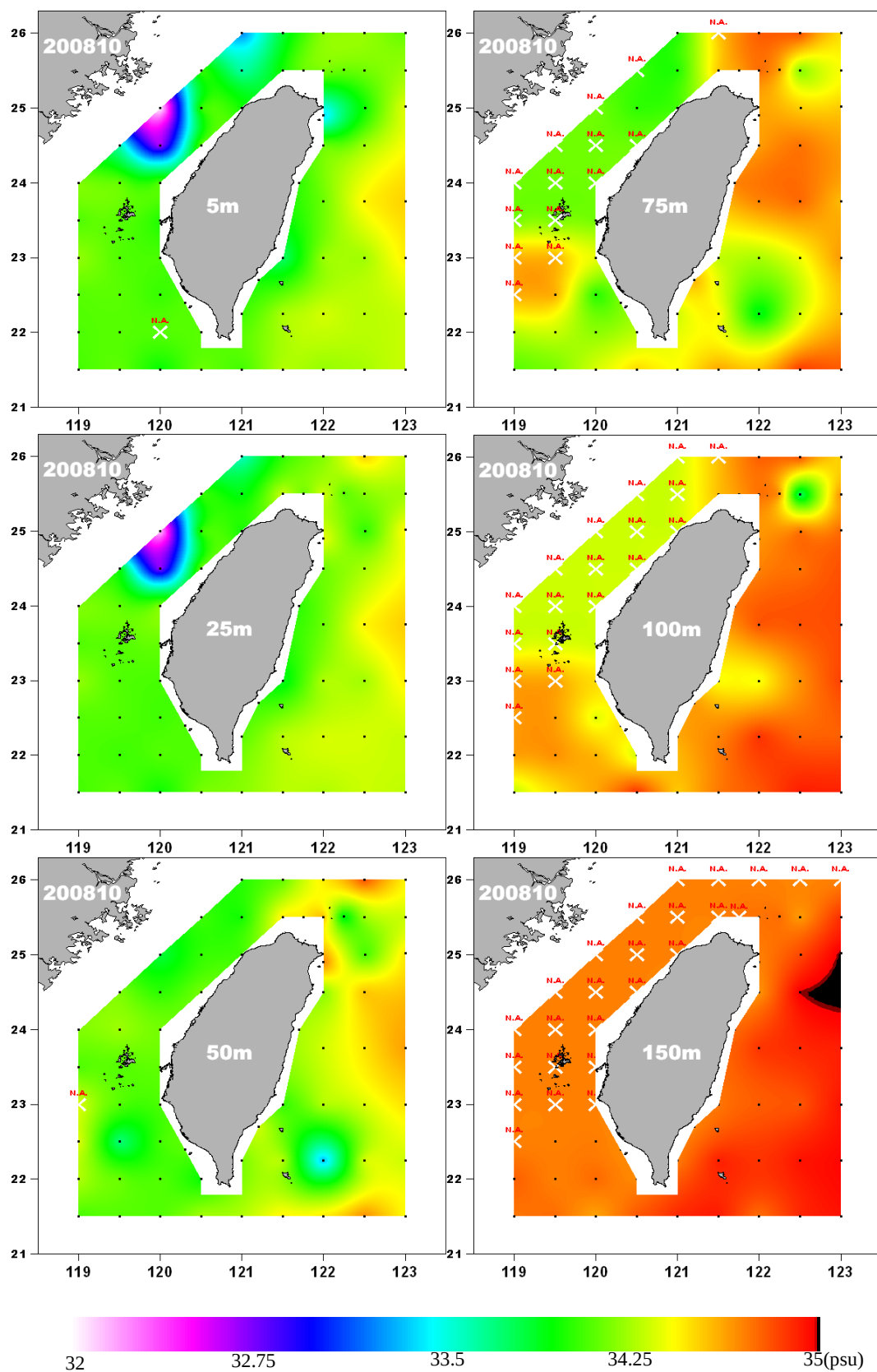
圖 12. 2008-10-14 航次鹽度分布 Fig. 12. Salinity distribution in Oct. 2008.
