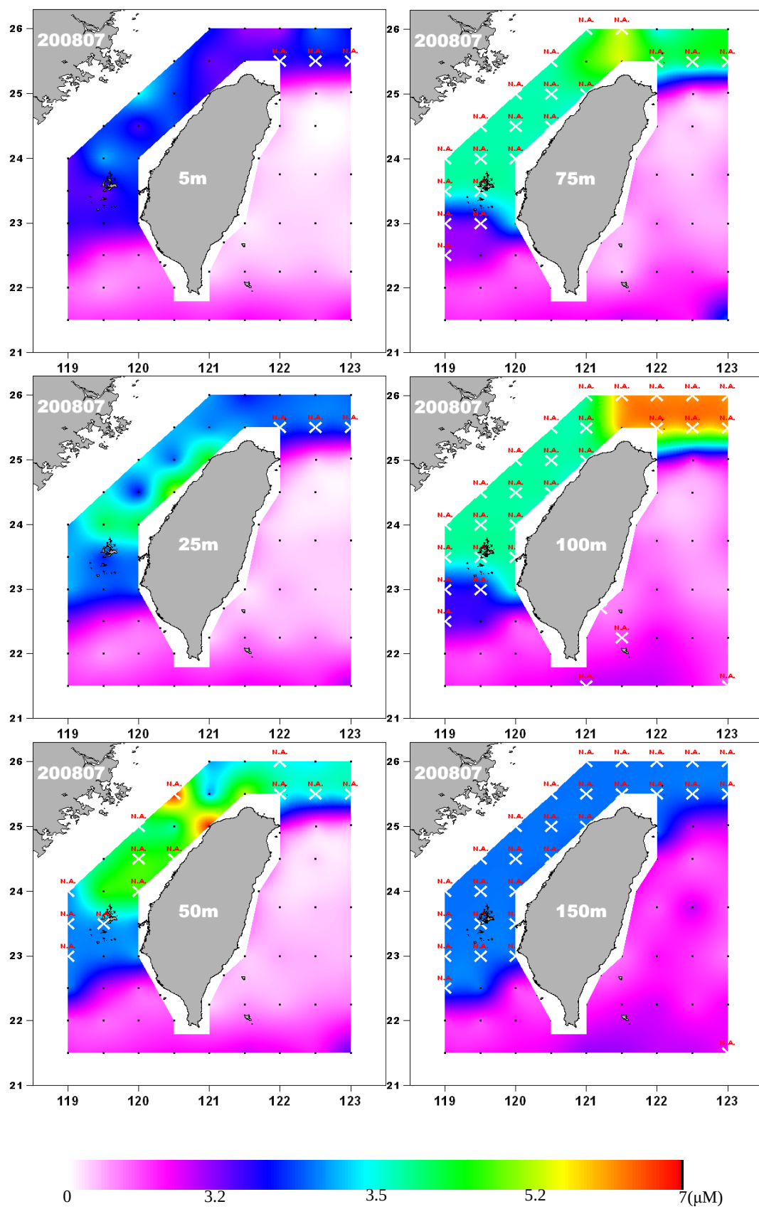
圖 15. 2008-07-03 航次硝酸鹽(NO 3 )濃度分布 Fig. 15. Nitrate (NO 3 ) distribution in Jul. 2008.
