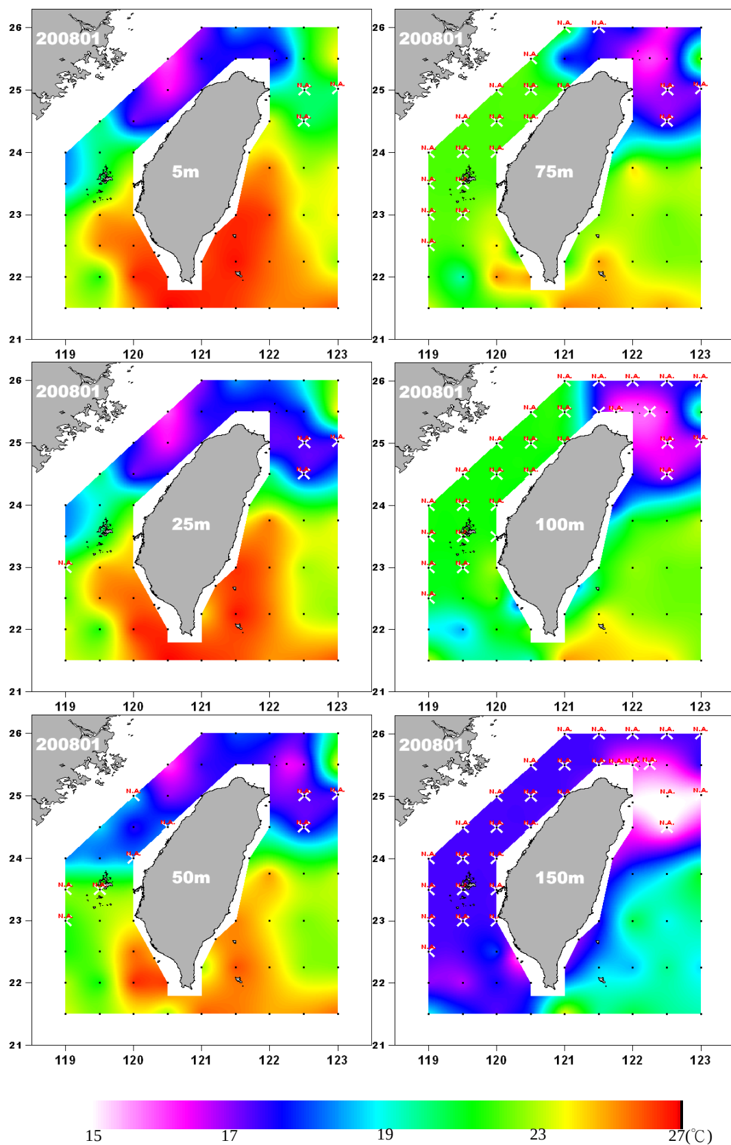
圖 5. 2008-01-04 航次水溫分布 Fig. 5. Temperature distribution in Jan. 2008.
