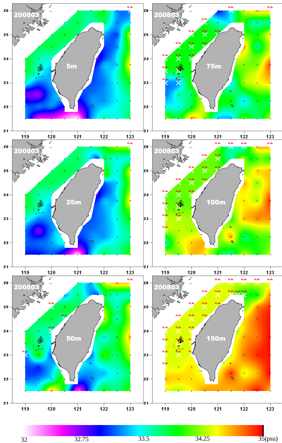
圖 10. 2008-03-13 航次鹽度分布 Fig. 10. Salinity distribution in Mar. 2008.
