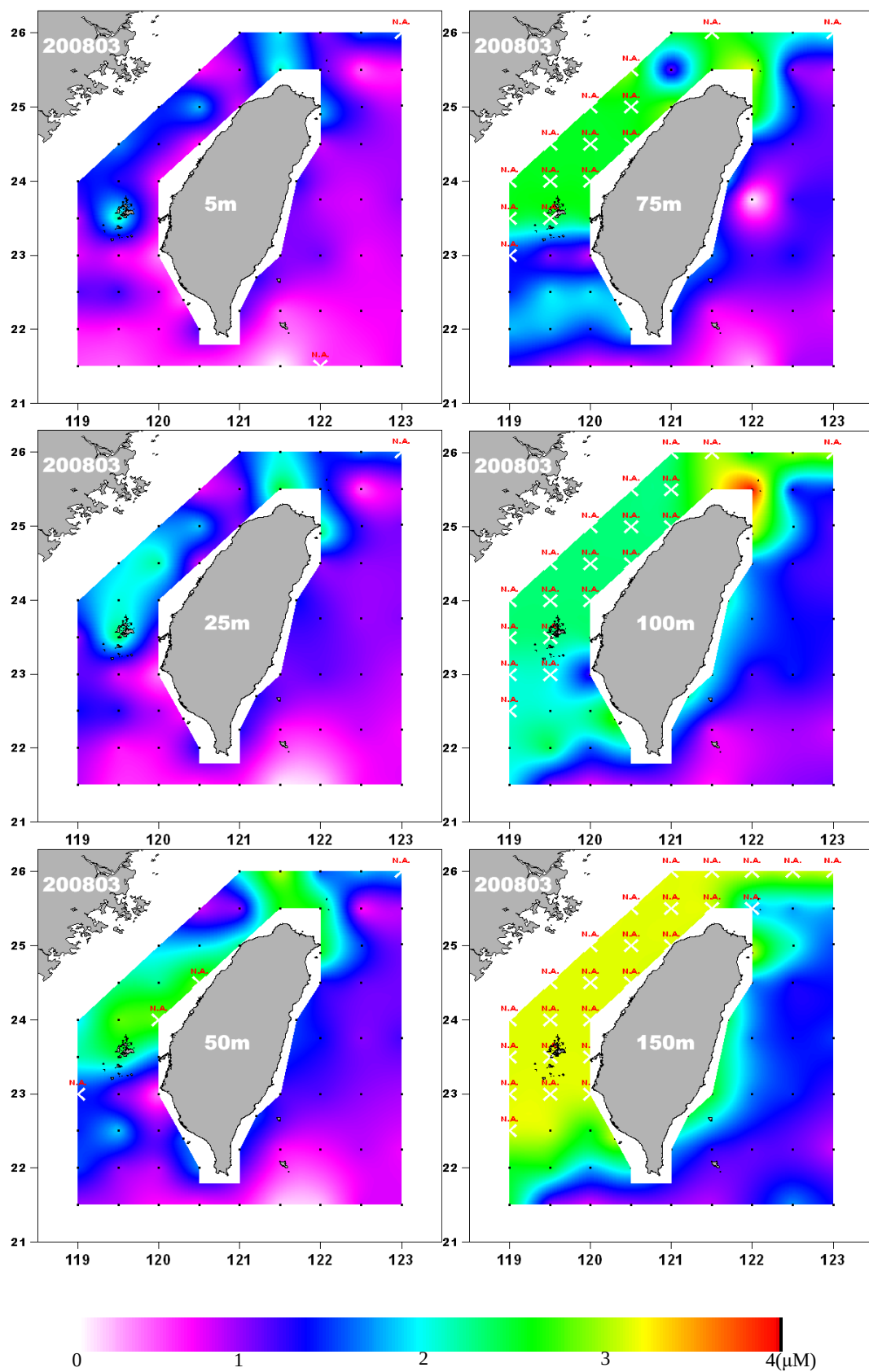
圖 14. 2008-03-13 航次硝酸鹽(NO 3 )濃度分布 Fig. 14. Nitrate (NO 3 ) distribution in Mar. 2008.
