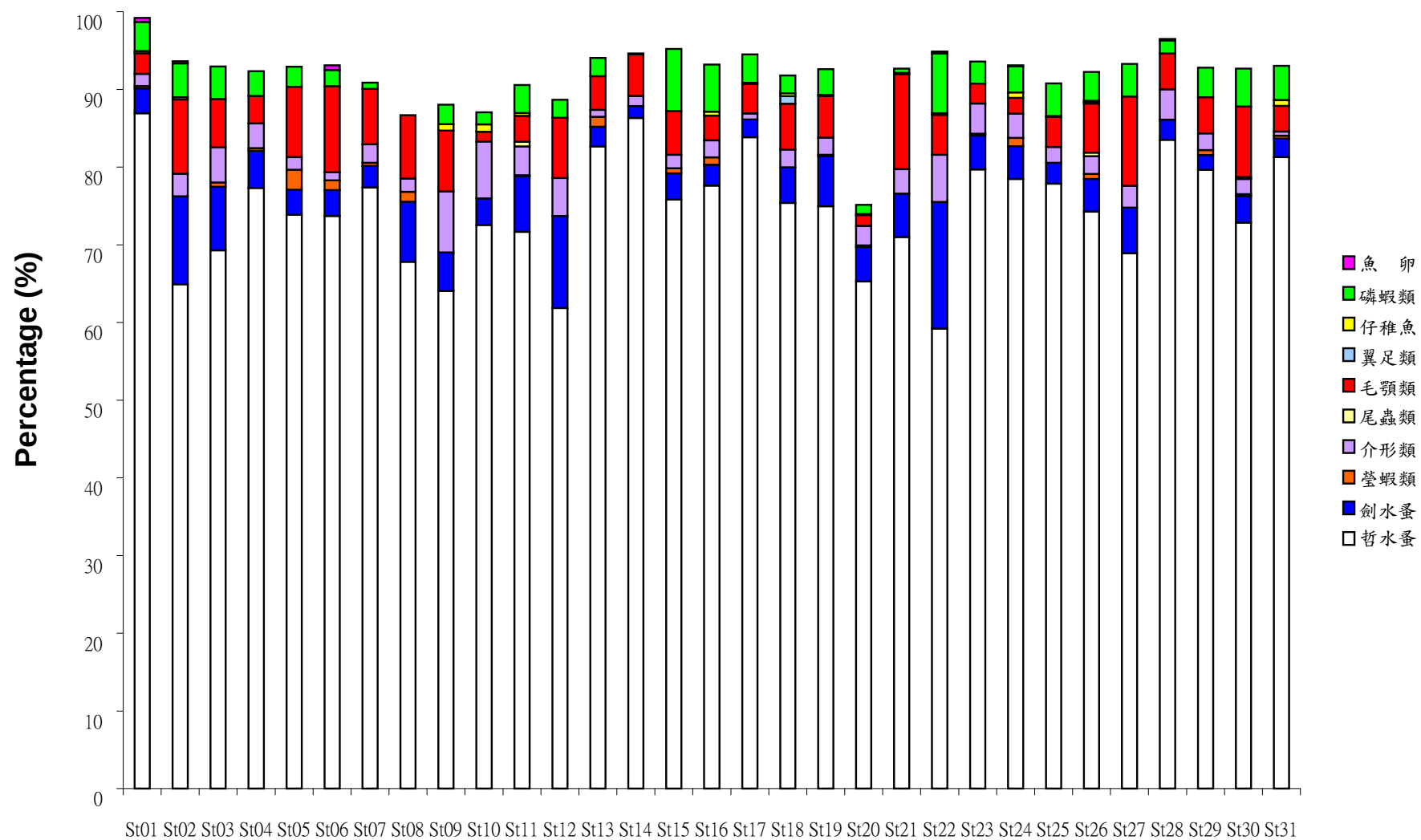
圖 34. 2008-03-13 航次浮游動物優勢大類出現百分率
