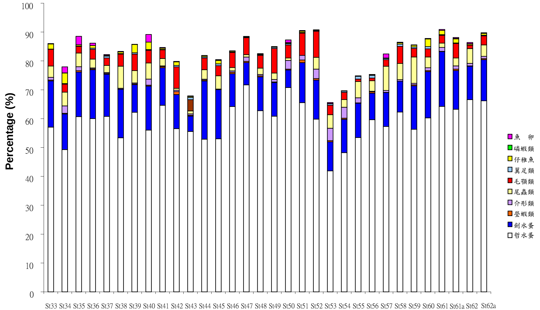
圖 39. 2008-10-14 航次浮游動物優勢大類出現百分率
