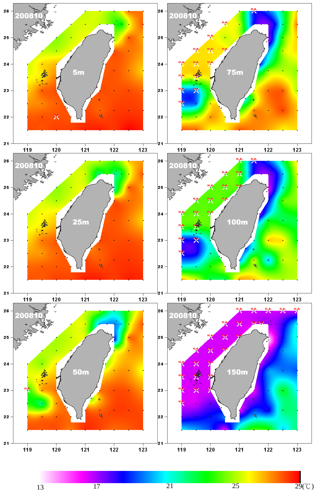
圖 8. 2008-10-14 航次水溫分布 Fig. 8. Temperature distribution in Oct. 2008.
