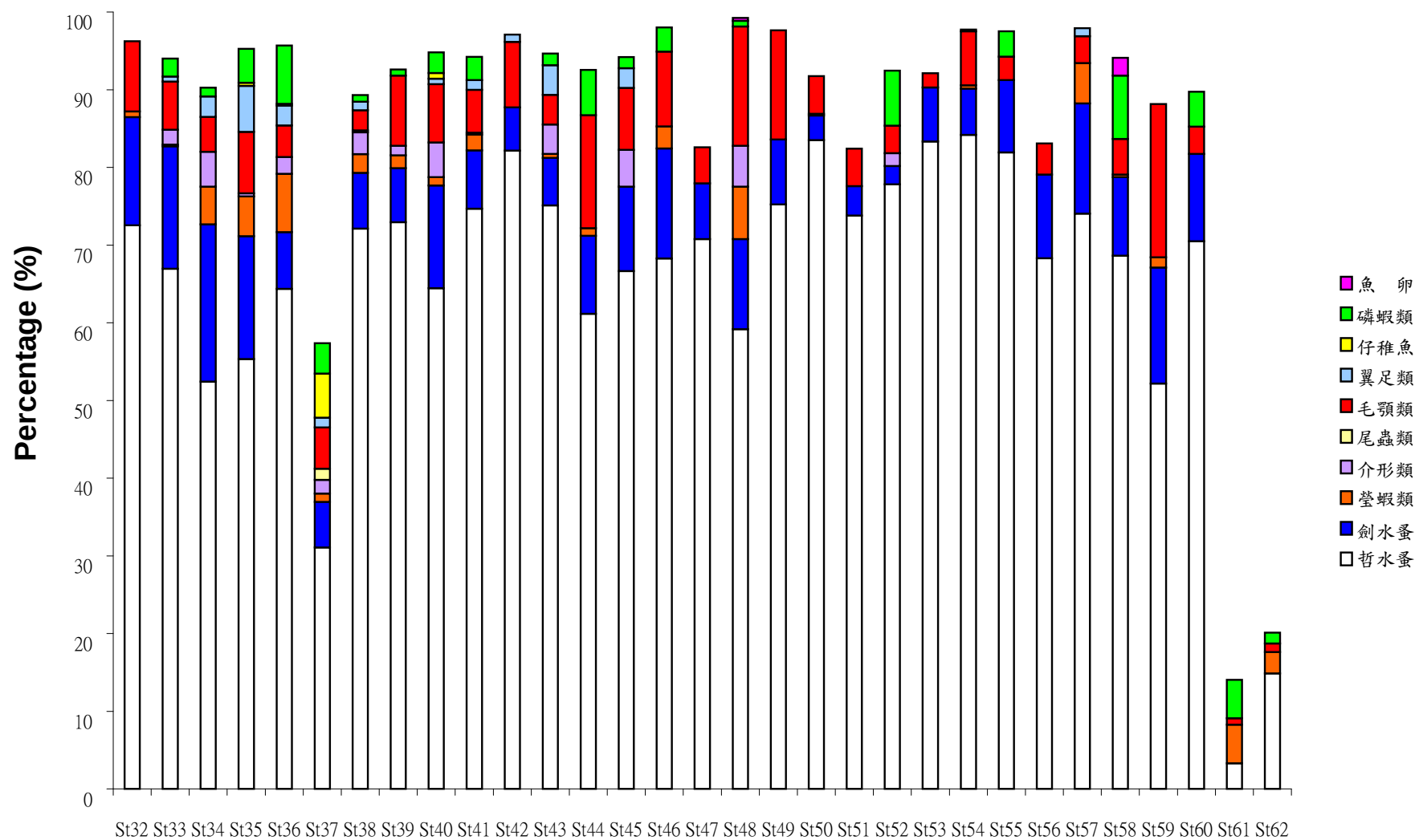
圖 37. 2008-07-03 航次浮游動物優勢大類出現百分率
