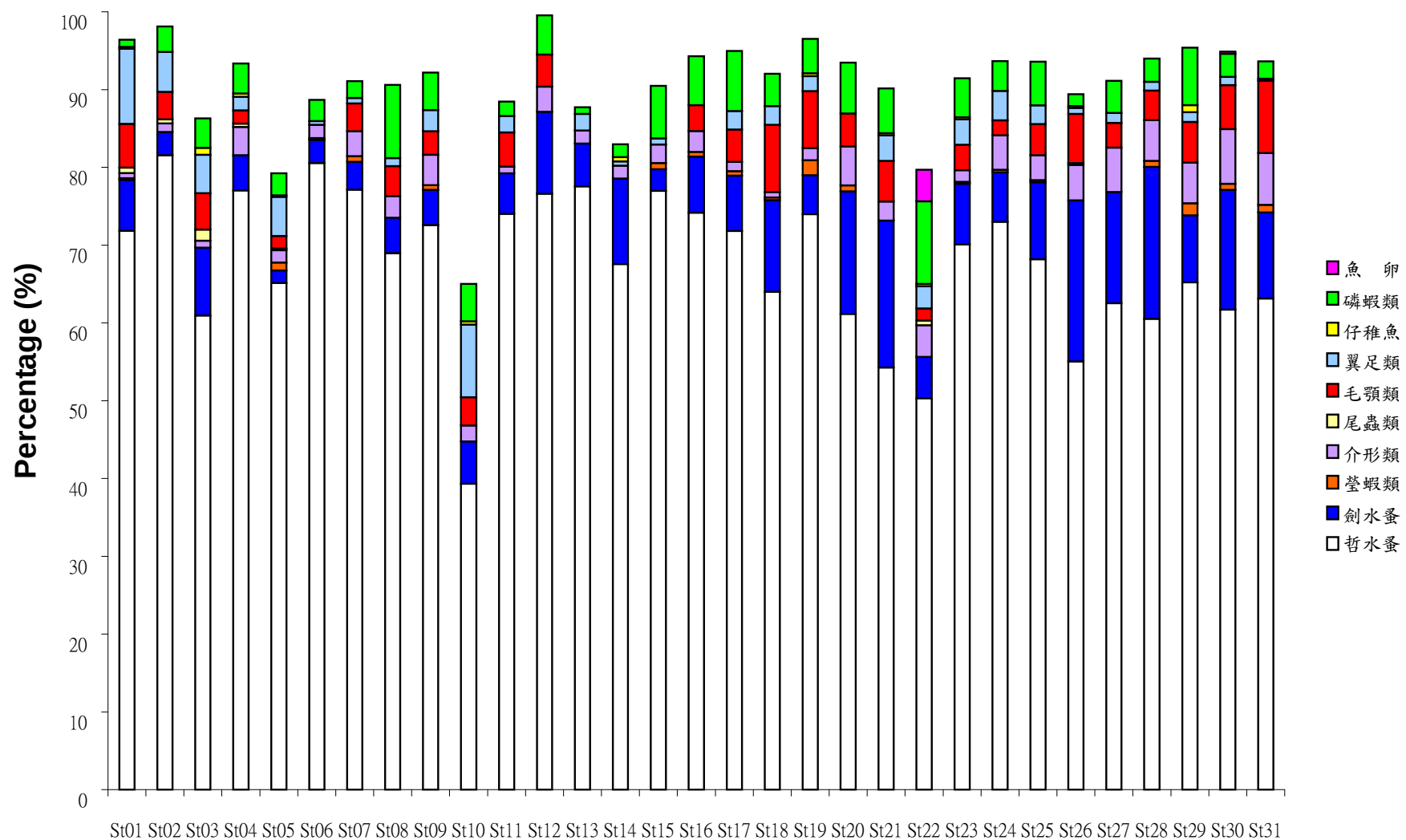
圖 36. 2008-07-03 航次浮游動物優勢大類出現百分率
