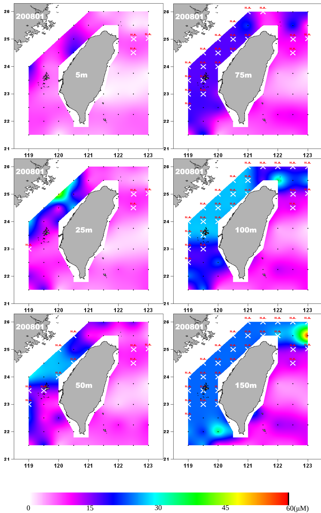
圖 21. 2008-01-04 航次矽酸鹽( \text{SiO}_4 )濃度分布 Fig. 21. Silicate ( \text{SiO}_4 ) distribution in Jan. 2008.
