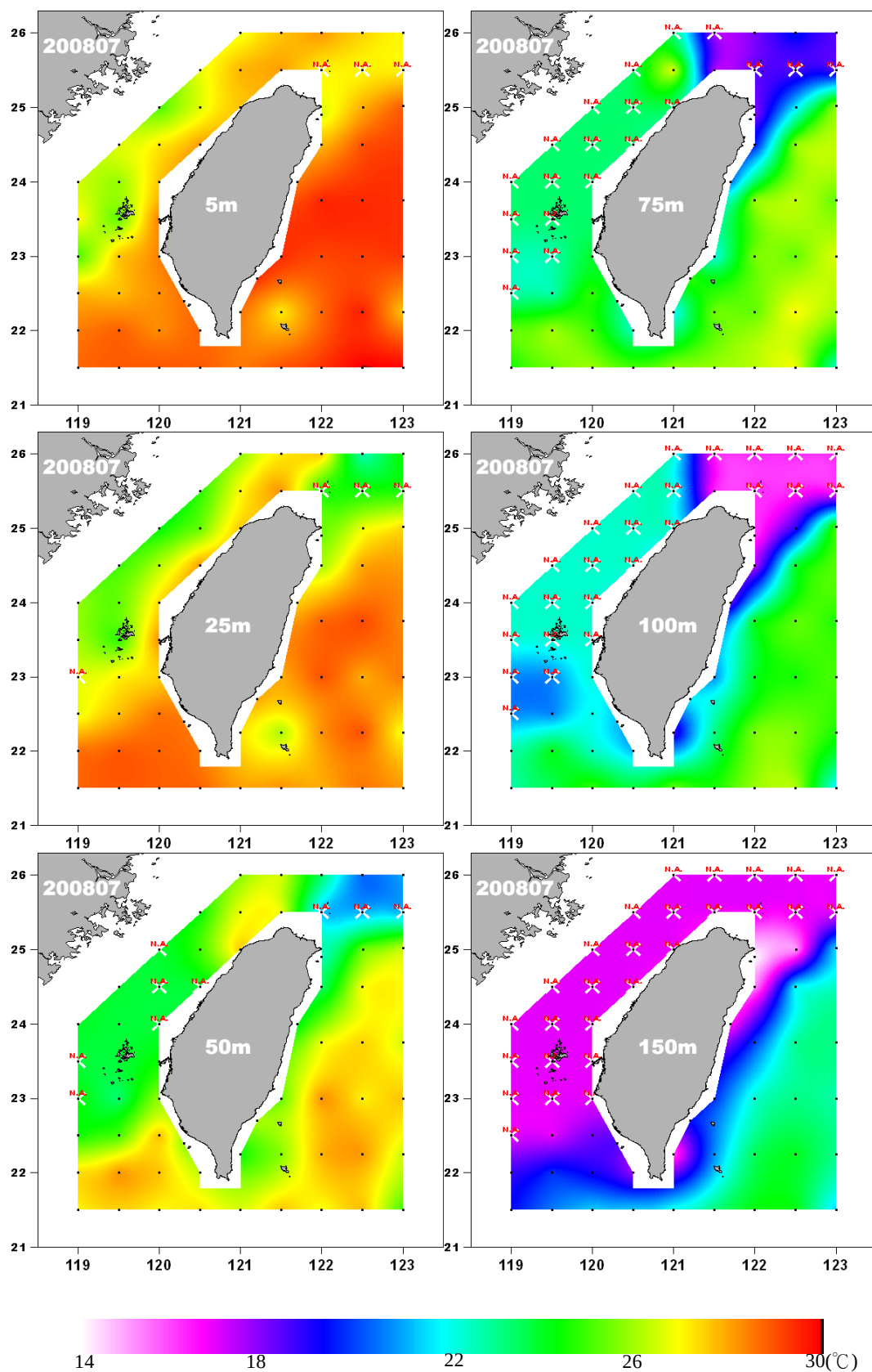
圖 7. 2008-07-03 航次水溫分布 Fig. 7. Temperature distribution in Jul. 2008.
