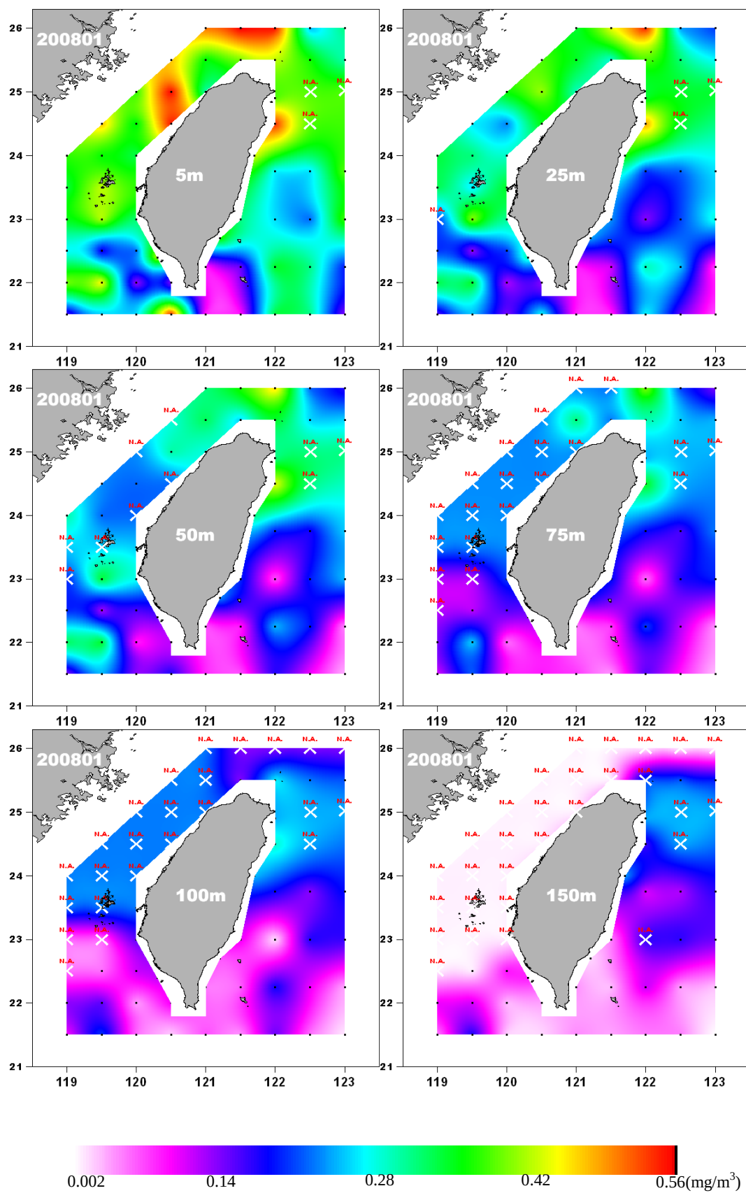
圖 25. 2008-01-04 航次葉綠素甲(chl-a)濃度分布 Fig. 25. chlorophyll(chl-a) distribution in Jan. 2008.
