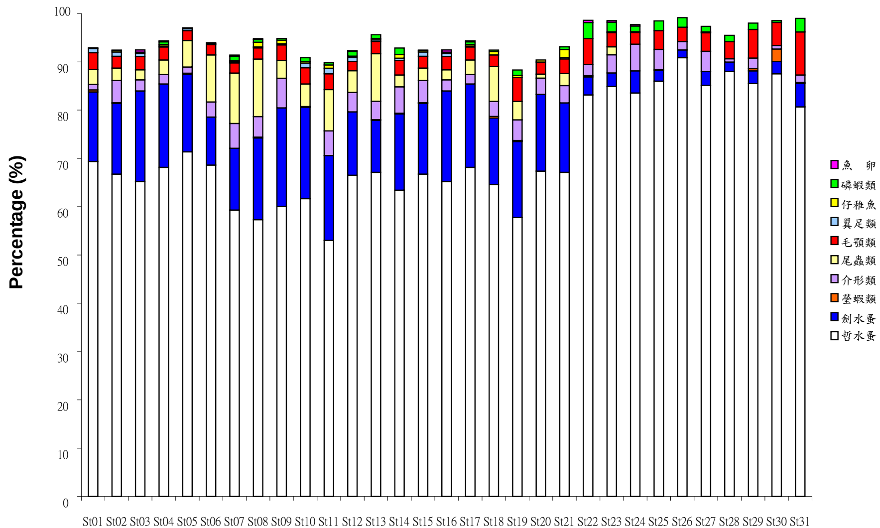
圖 32. 2008-01-04 航次浮游動物優勢大類出現百分率
