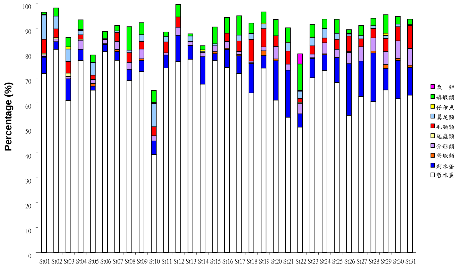
圖 38. 2008-10-14 航次浮游動物優勢大類出現百分率
