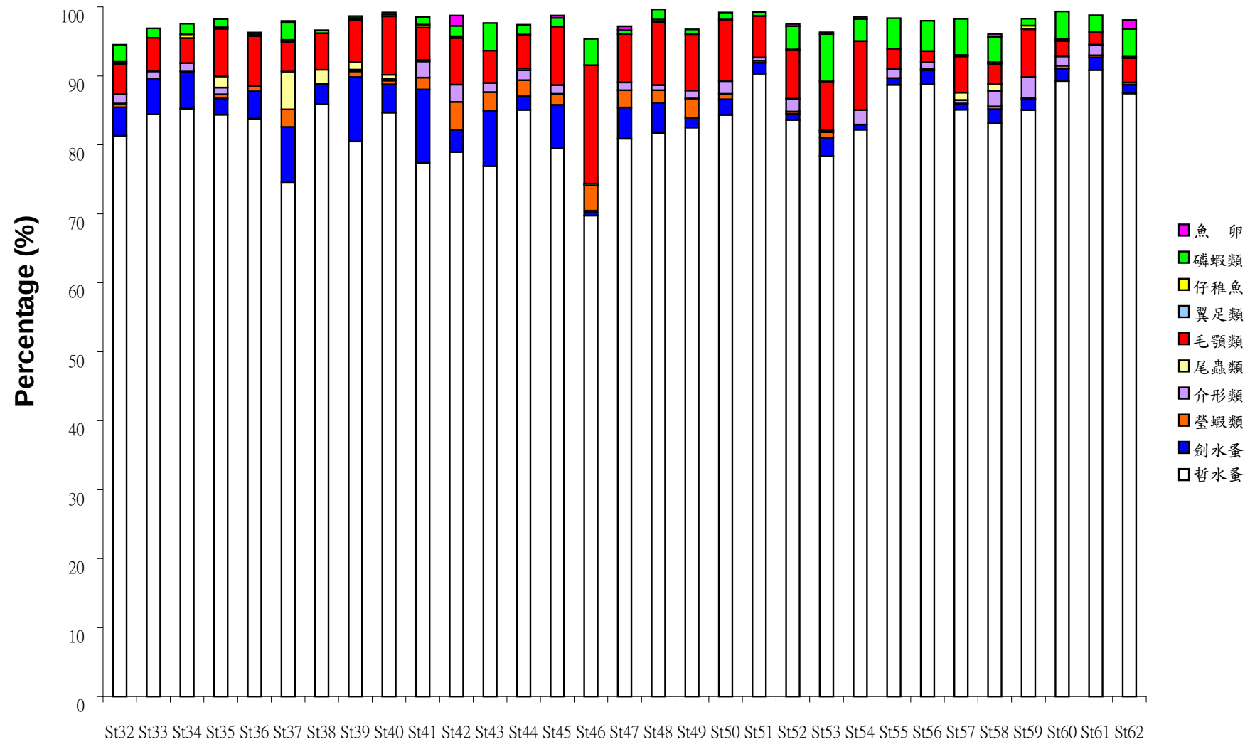
圖 33. 2008-01-04 航次浮游動物優勢大類出現百分率
