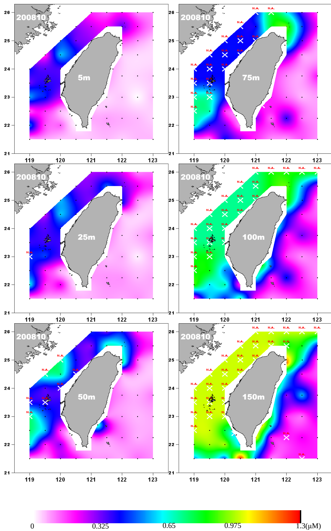
圖 20. 2008-10-14 航次磷酸鹽( \text{PO}_4 )濃度分布 Fig. 20. Phosphate ( \text{PO}_4 ) distribution in Oct. 2008.
