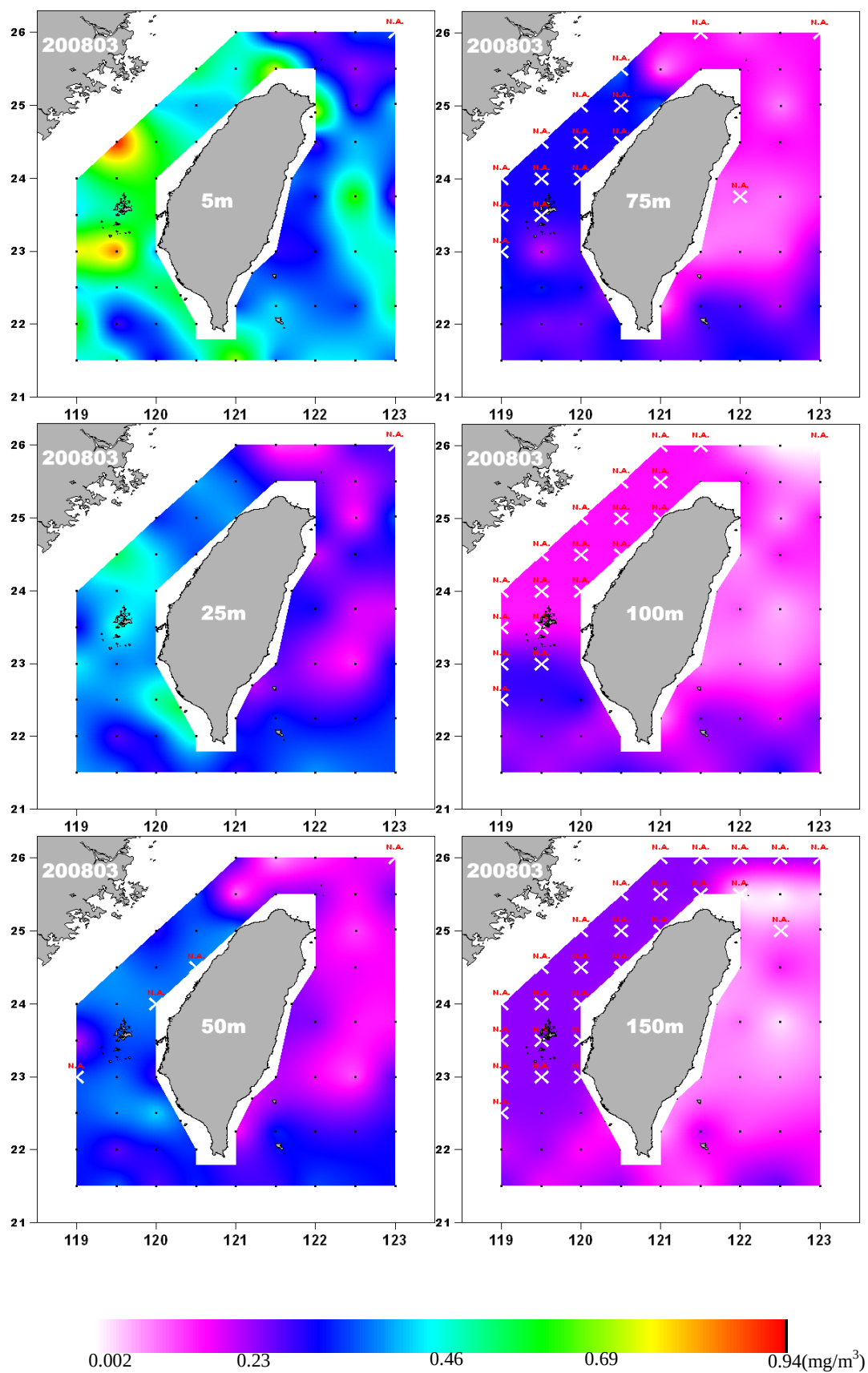
圖 26. 2008-03-13 航次葉綠素甲(chl- a )濃度分布 Fig. 26. chlorophyll(chl- a ) distribution in Mar. 2008.
