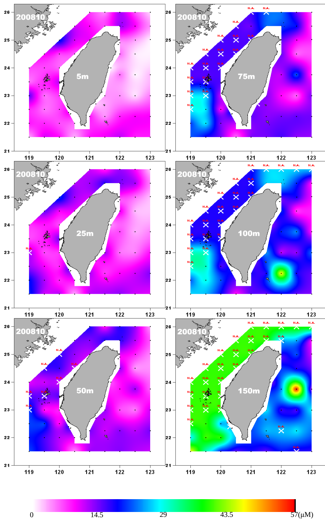
圖 24. 2008-10-14 航次矽酸鹽( \text{SiO}_4 )濃度分布 Fig. 24. Silicate ( \text{SiO}_4 ) distribution in Oct. 2008.
