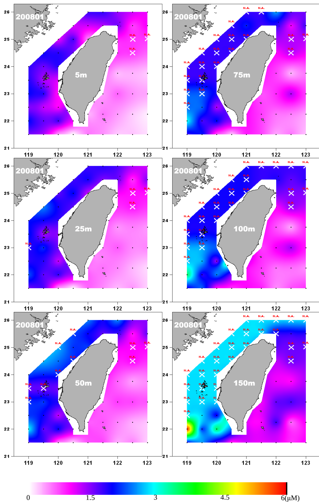
圖 13. 2008-01-04 航次硝酸鹽( \text{NO}_3 )濃度分布 Fig. 13. Nitrate ( \text{NO}_3 ) distribution in Jan. 2008.
