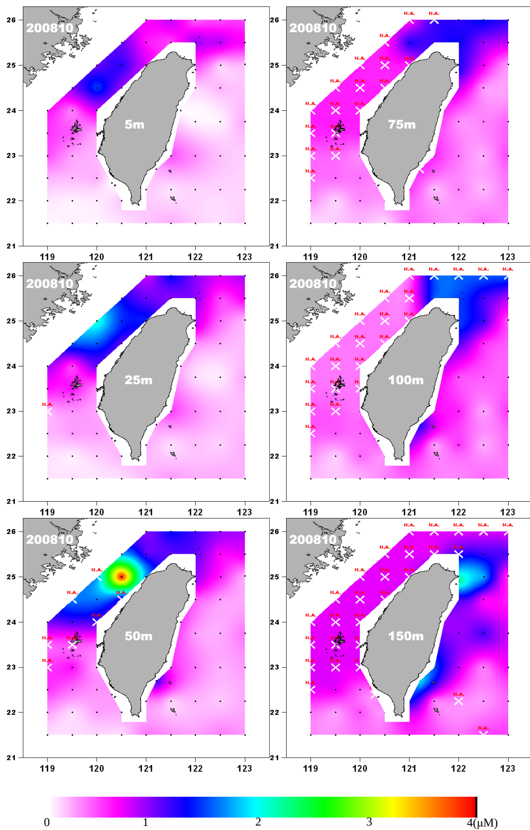
圖 16. 2008-10-14 航次硝酸鹽( \text{NO}_3 )濃度分布 Fig. 16. Nitrate ( \text{NO}_3 ) distribution in Oct. 2008.
