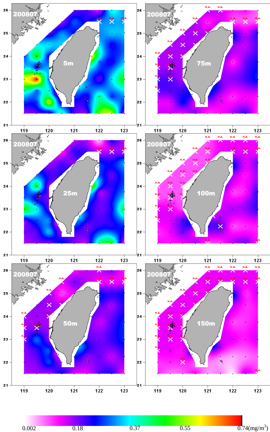
圖 27. 2008-07-03 航次葉綠素甲(chl-a)濃度分布 Fig. 27. chlorophyll(chl-a) distribution in Jul. 2008.
