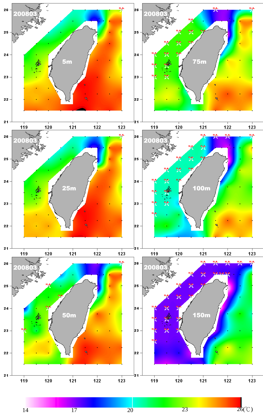
圖 6. 2008-03-13 航次水溫分布 Fig. 6. Temperature distribution in Mar. 2008.
