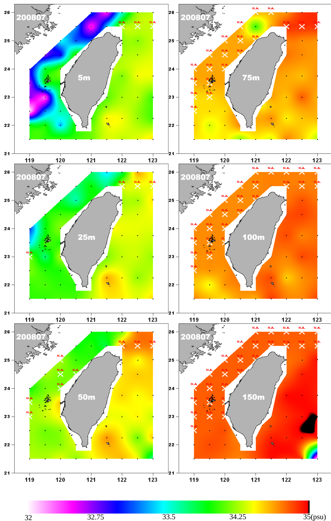
圖 11. 2008-07-03 航次鹽度分布 Fig. 11. Salinity distribution in Jul. 2008.
