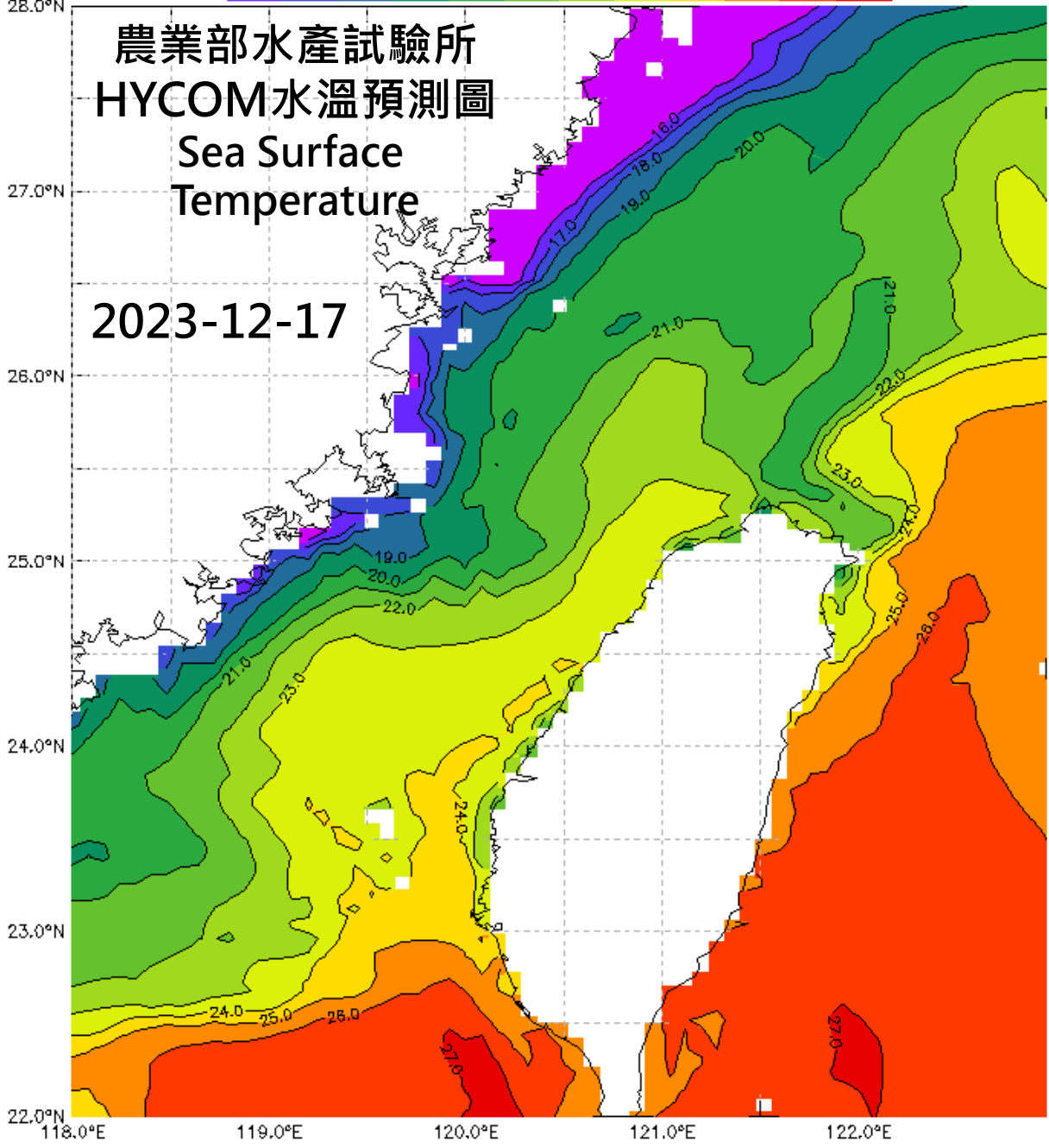
HYCOM模式-水溫預測圖 2023-12-18製圖
