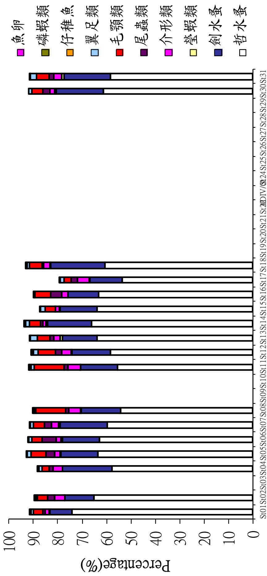
圖 35. 2014 年 10 月航次浮游動物優勢大類出現百分率 Fig. 35. Percentage of the composition of zooplankton in Oct. 2014.
