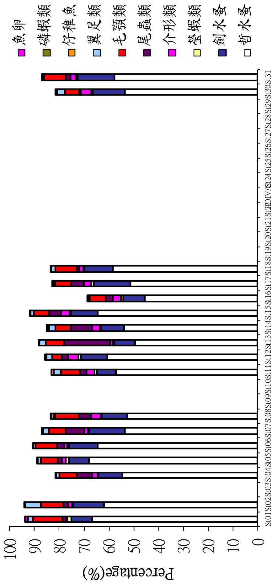
圖 33. 2014 年 8 月航次浮游動物優勢大類出現百分率 Fig. 33. Percentage of the composition of zooplankton in Aug. 2014.
